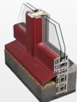
Warmtegeoptimeerde en winterharde vloeraansluitingen met meerkamerprofielen
