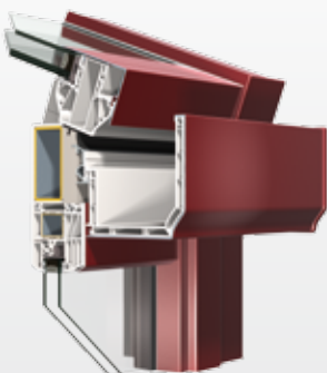
De goot met prima warmte- en geluidsisolatie
